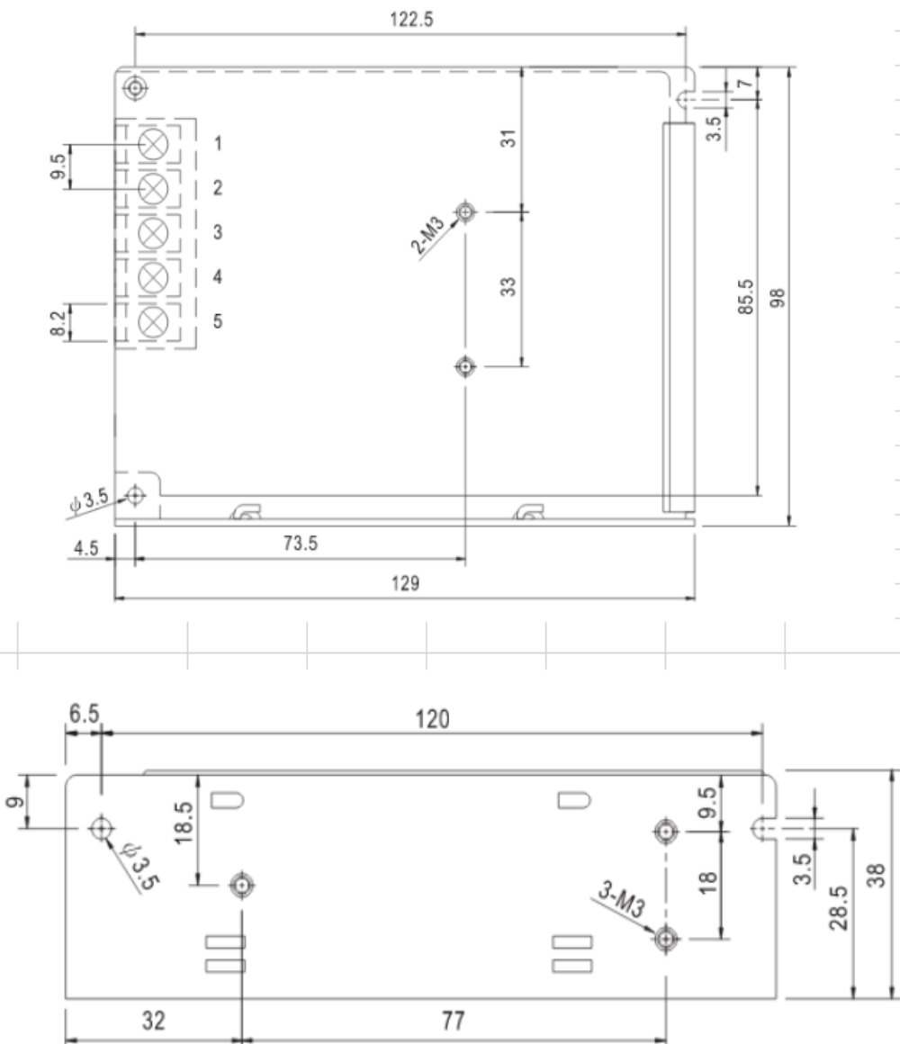
■ 机构尺寸
